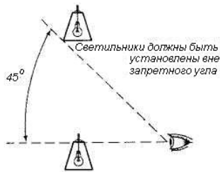
Рис. 4.3. Схема установки светильников
