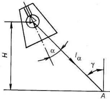
Рис. 4.4. Схема расчета точечным методом
