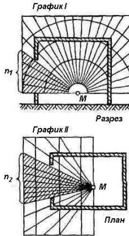
Рис. 4.5. Схема для расчета естественного освещения по методу А. М. Данилюка
