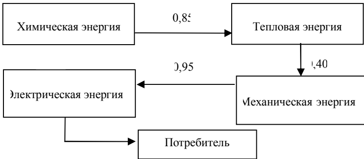
Рис.1.2. Схема получения электрической энергии на ТЭС
