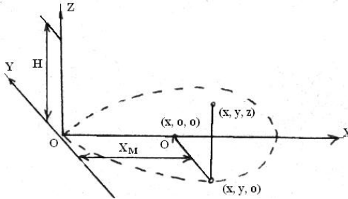
Рис. 4.1. Схема рассеивания веществ в атмосфере: O' – центральная точка рассеивания по оси факела; OX – ось факела; (x, y, z) – координаты точек, в которых определяют концентрацию вредных веществ
